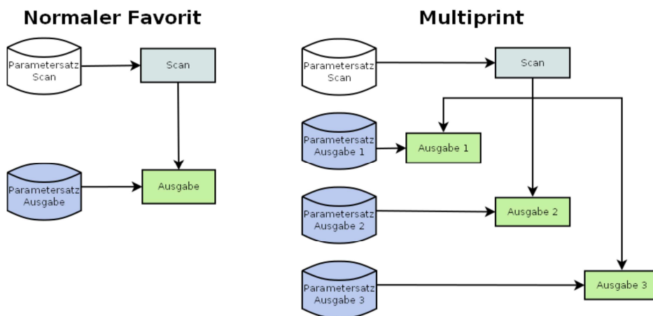
Abbildung 5.37: Konzept Favorit – Multiprint
