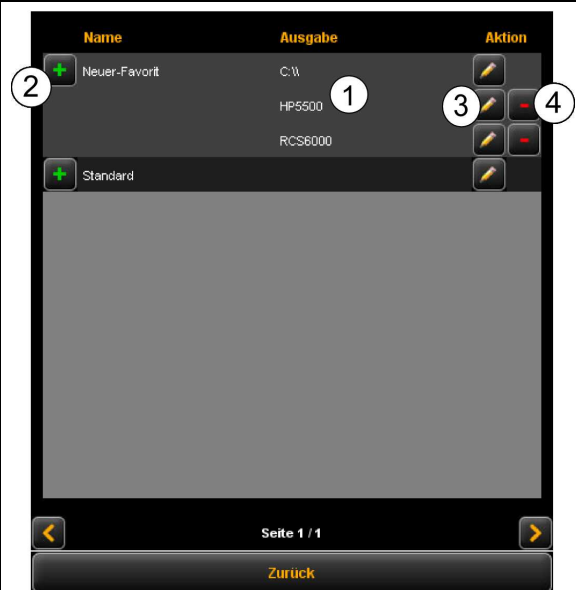
Abbildung 5.39: Multiprint Favoriten erstellen / bearbeiten
