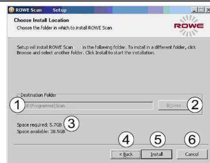
Abbildung 2.4: Auswahl des Zielverzeichnisses
